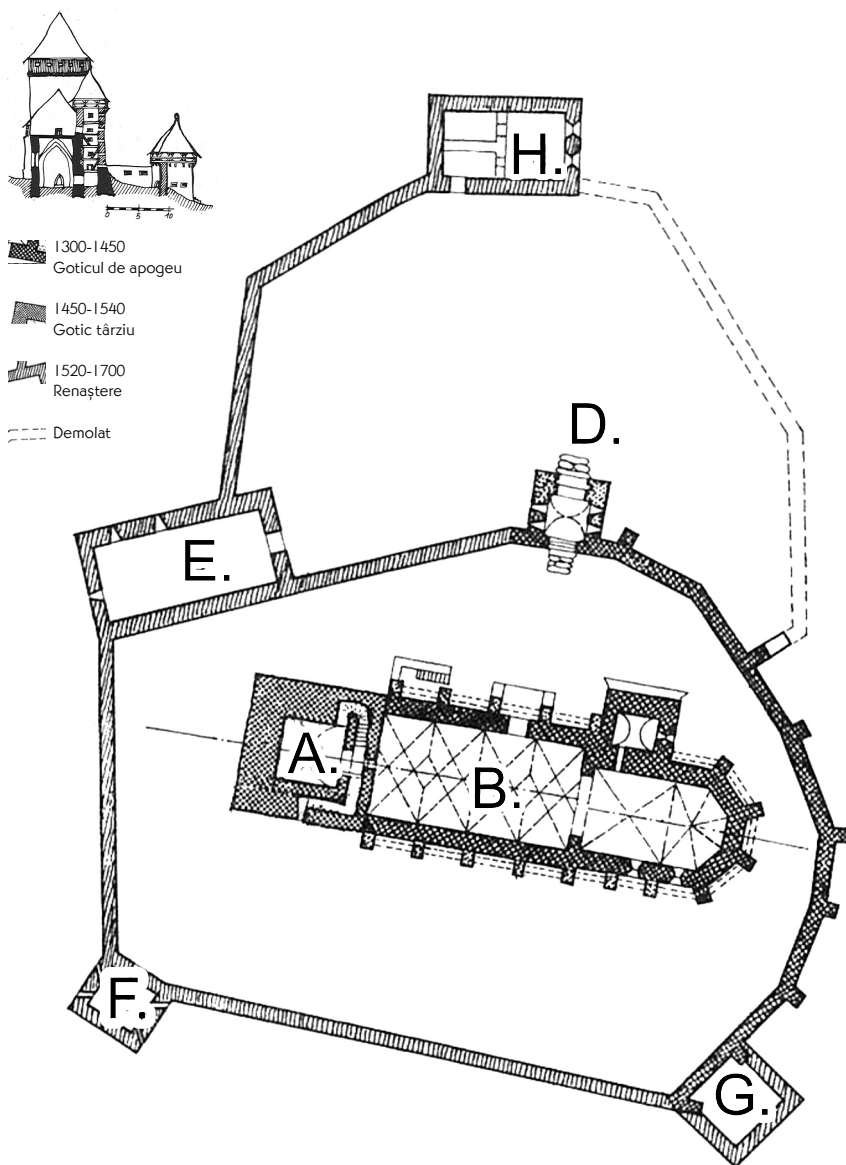
Fig. 2. Planul bisericii fortificate din Iacobeni / Agnita.
